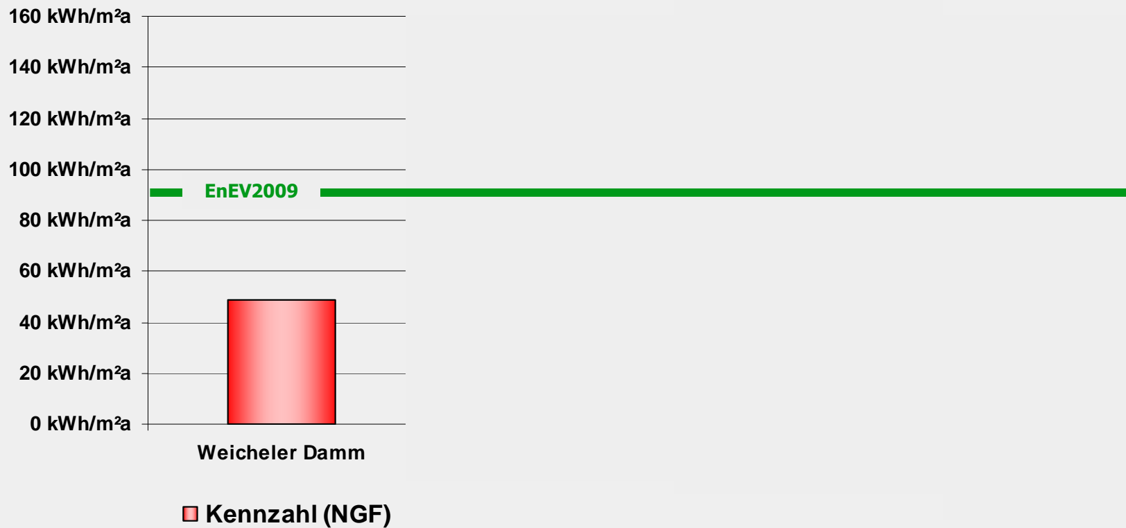
Heizenergie-Kennzahl (NGF)
