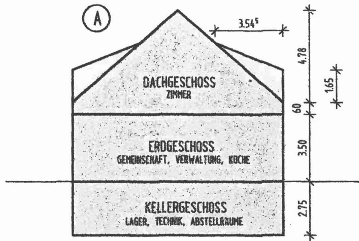
SNITT 1:200
